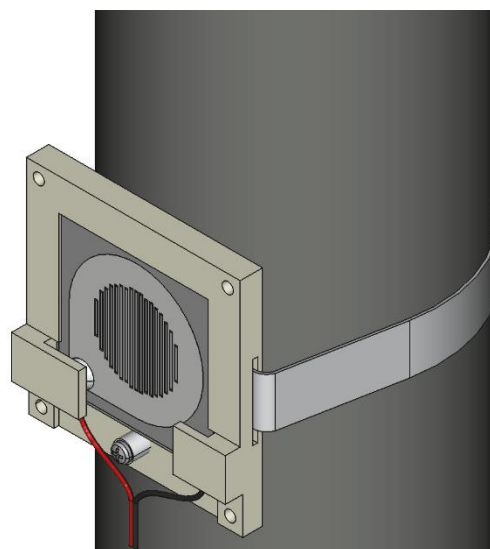
<円柱に設置>
